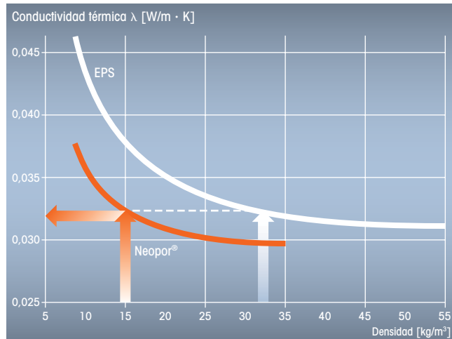
Conductividad térmica en función de la densidad. Neopor® en comparación con EPS blanco, medido según DIN EN 13 163.
